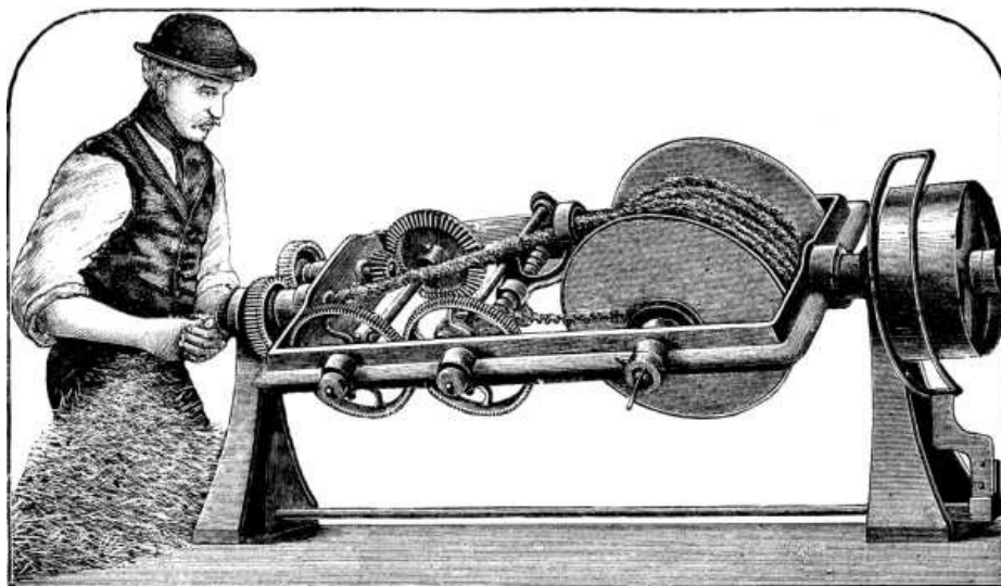
HAY ROPE MACHINE.
