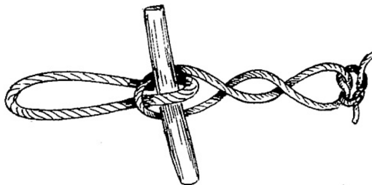
FIG. 144.—Rope buckle.
