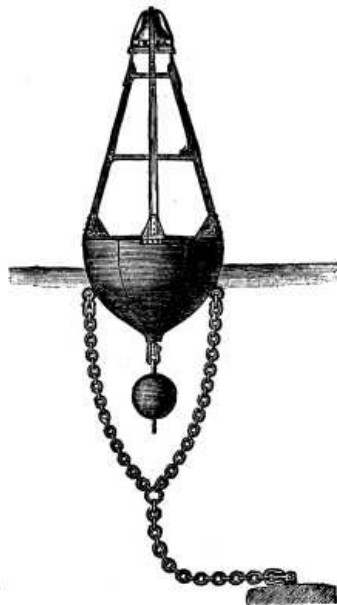
FIG. 2.—BROWN'S BELL BUOY.
