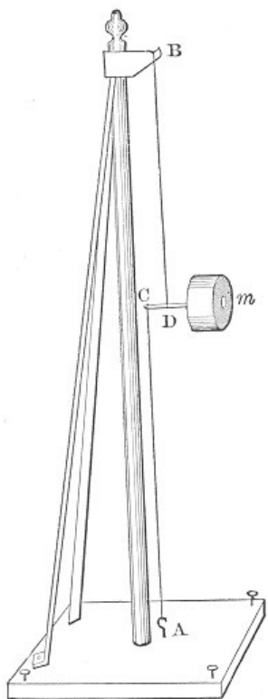
Fig. 82.—Horizontal Pendulum.
