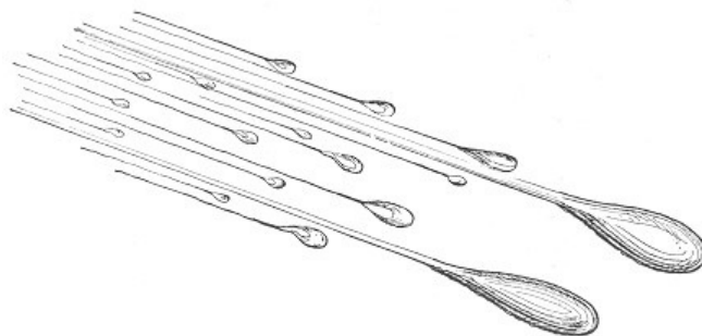
Fig. 49.—Bolides.
