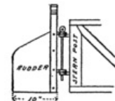
Fig. 114. The Rudder Hinge.
