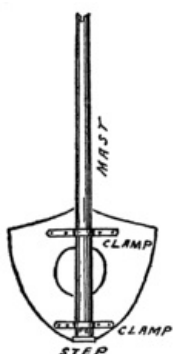
Fig. 117. The Mast Step.
