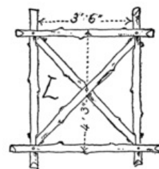
Fig. 316. L Frame (make two).
