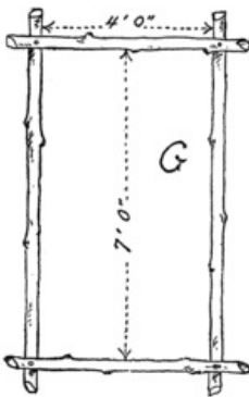
Fig. 311. G Frame (make two).
