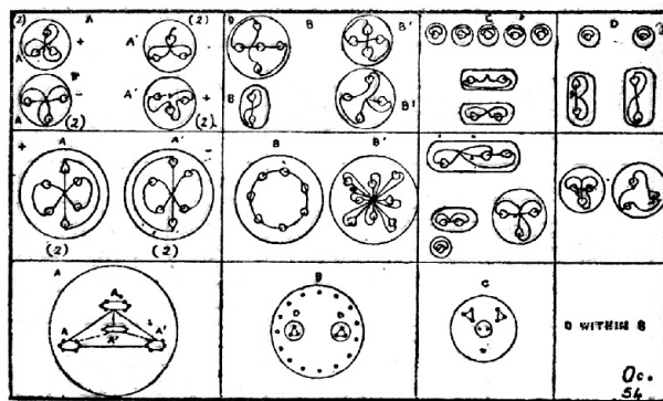
SODIUM (Plate VI, 2).
