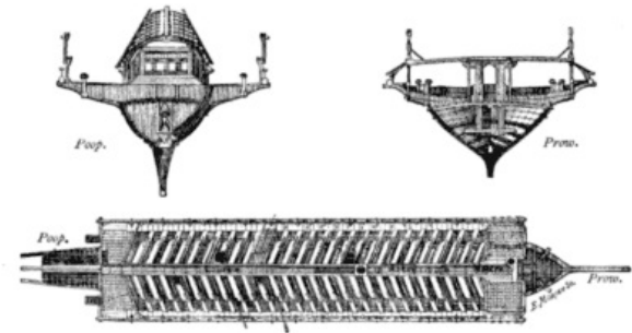
PLAN AND SECTIONS OF A GALLEY. ( Jurien de la Gravière. )
