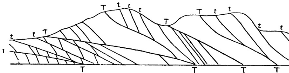
FIG. 78.—Diagram of Thrust-planes.
