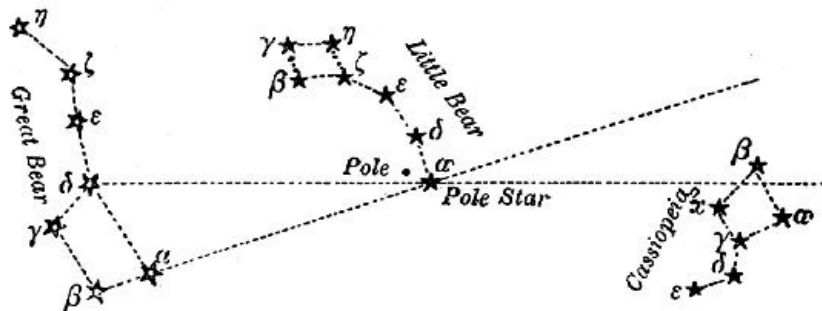
FIG. 5.—To find Cassiopeia.
