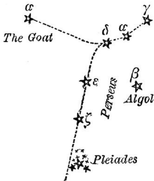
FIG. 7.—Perseus, the Pleiades, Capella.
