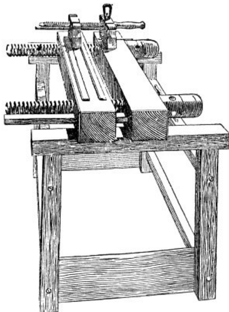
Fig. 46.—Lying or Cutting Press
