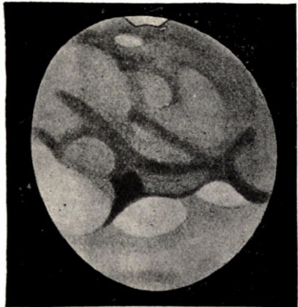
Fig. 52.—Drawing of Mars (August 16th, 1894).
