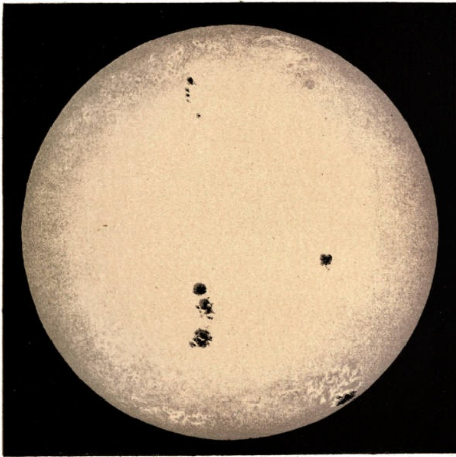
PLATE A. THE SUN.
