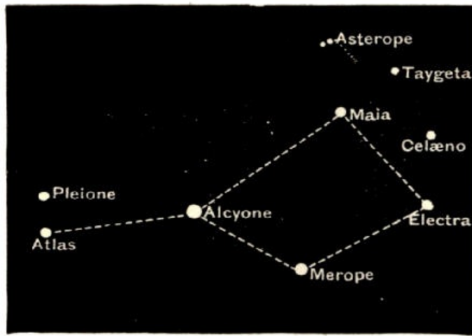
Fig. 84.—The Pleiades.
