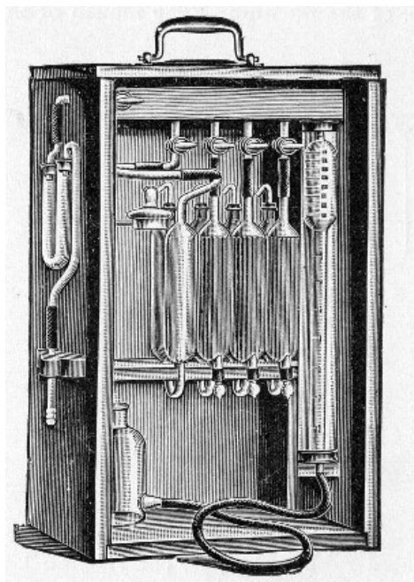
Fig. 154.—Orsat-Lunge gas analysis apparatus.
