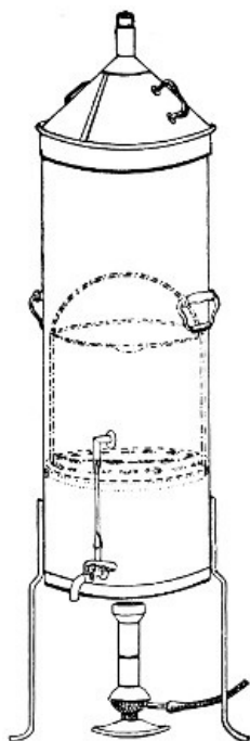
Fig. 28.—Koch's steriliser.
