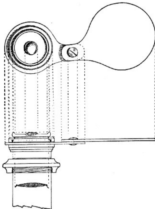
Fig. 49.—Eye shade.
