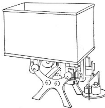
Fig. 166.—Rabbit scales.
