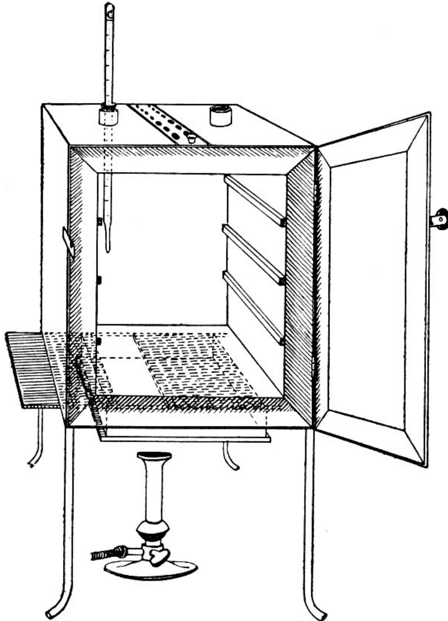
Fig. 26.—Hot-air oven.
