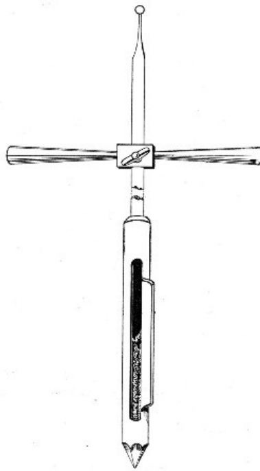
Fig. 218.—Fraenkel's borer.
