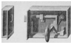
SERRURE APPELÉE BEC DE CANE.—C'est la serrure la plus simple. Il suffit, pour la fermer, de pousser la porte; le ressort, qu'on voit à droite, la maintient fermée.
