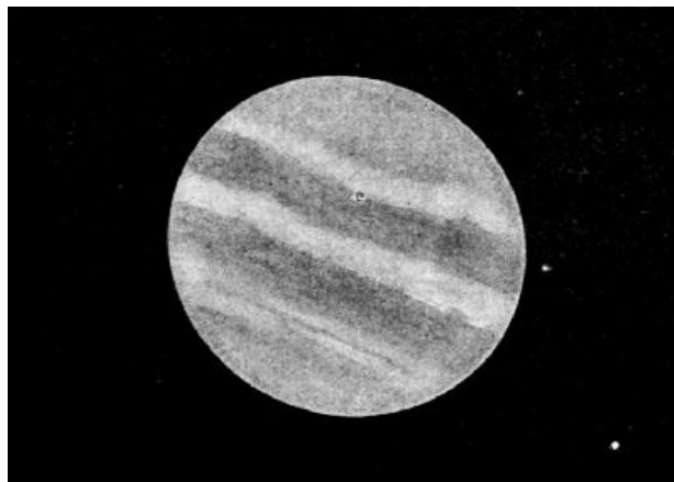
FIG. 72.—Jupiter.
