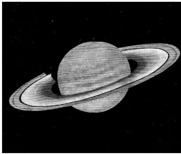
FIG. 81.—Saturn.
