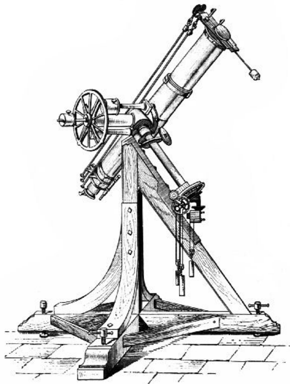
FIG. 92.—Heliometer.
