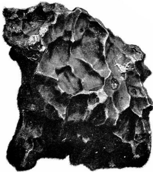
FIG. 95.—Meteorite.
