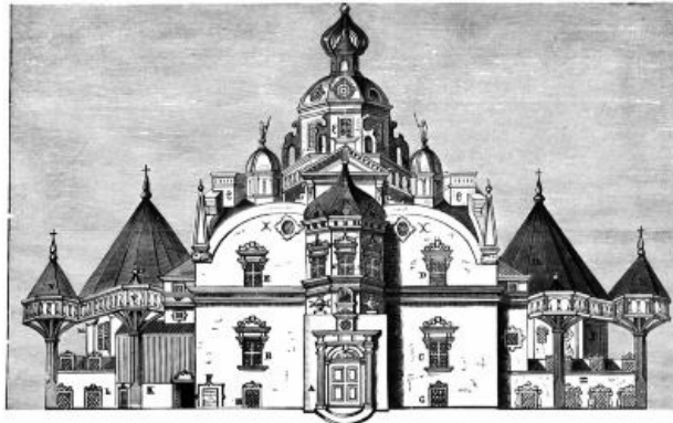
FIG. 20.—Uraniburg.
