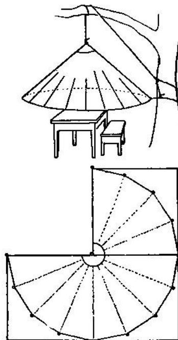
Fig. 11. Sibley awning
