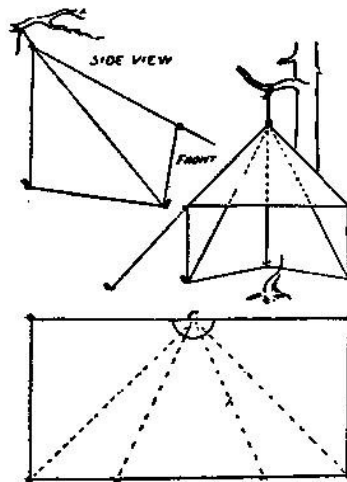
Fig. 5. The toque tent
