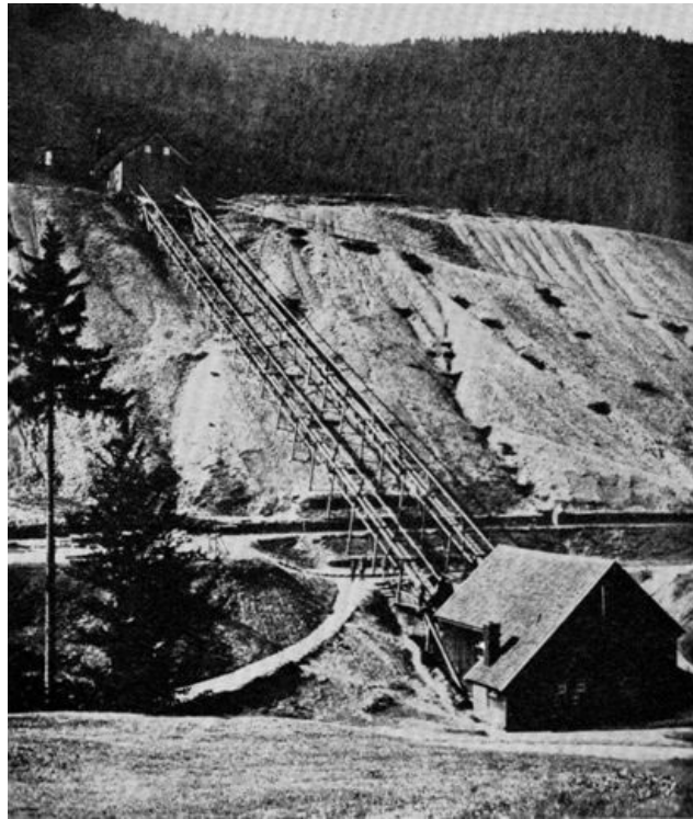
Figure 7.—FELDGESTANGE (STANGENKUNST) NEAR LAUTENTAL. From C. Matschoss, Technische Kulturdenkmal , Munich, 1932.
