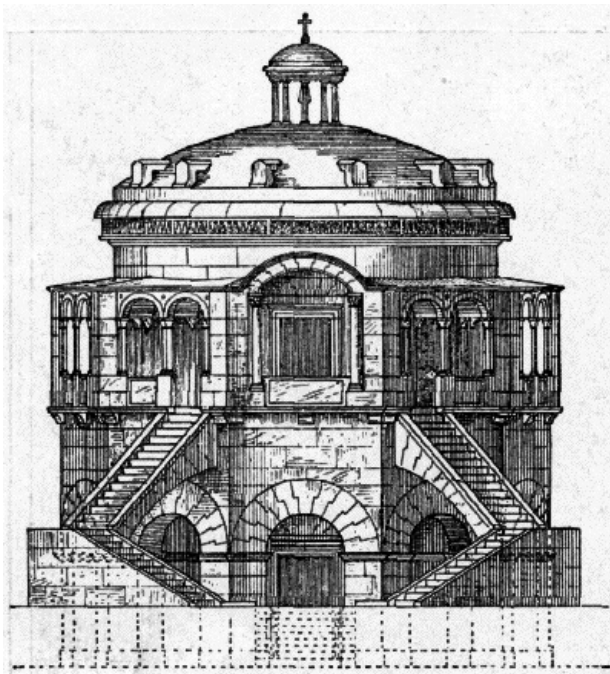
Bild 3. Das Grab des Theoderich, Rekonstruktion von Essenwein.
