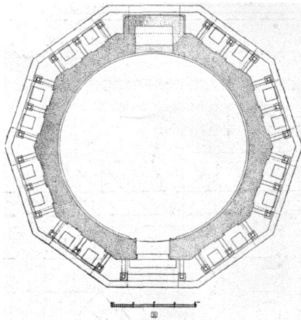
Bild 24. Grundriss des Obergeschosses, rekonstruiert von Bruno Schulz.
