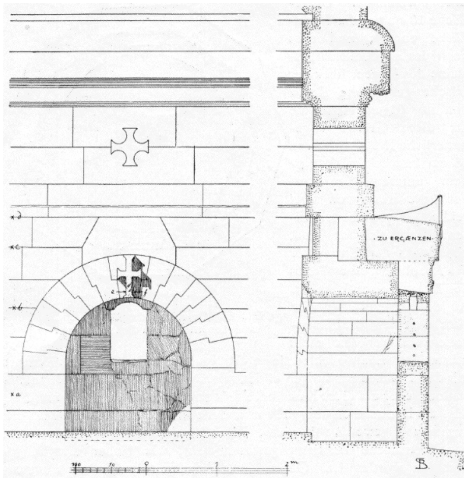
Bild 25. Die Nische in der Ostwand des Obergeschosses, Innenansicht und Schnitt. In den Höhen a, b, c, d und bei e und f eiserne Haften.
