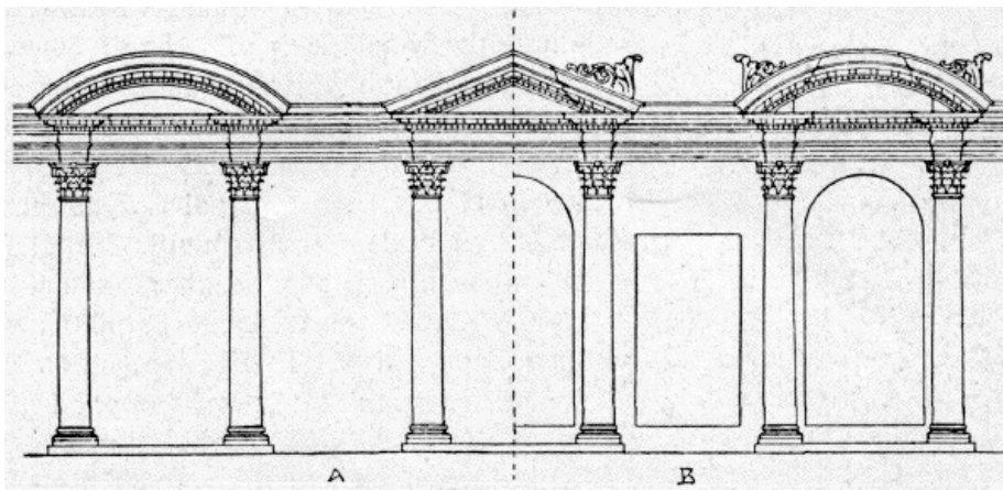
Bild 11. Schema einer Ädiculenreihe, in zwei Variationen.
