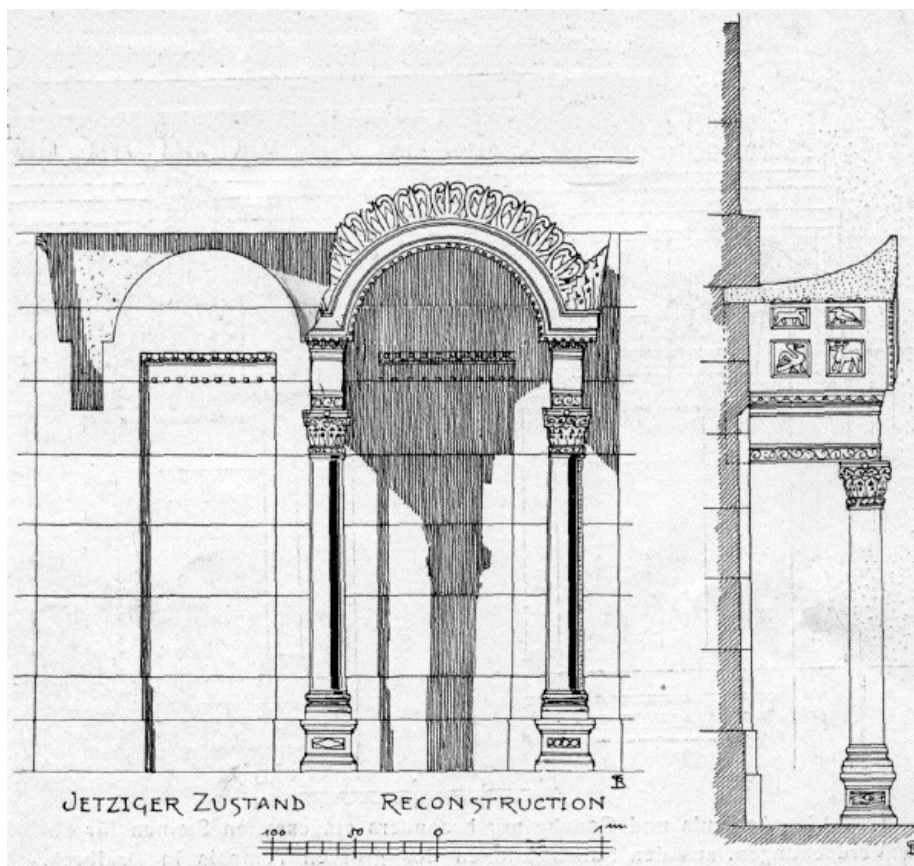
Bild 15. Die acht gleichen Wände des Obergeschosses.
