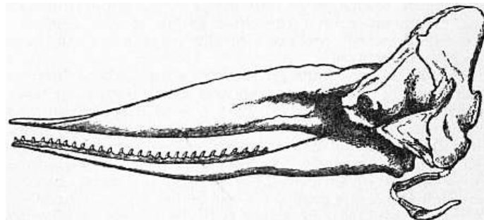
FIG. 2.—Skull of Sperm-Whale ( Physeter macrocephalus ).
