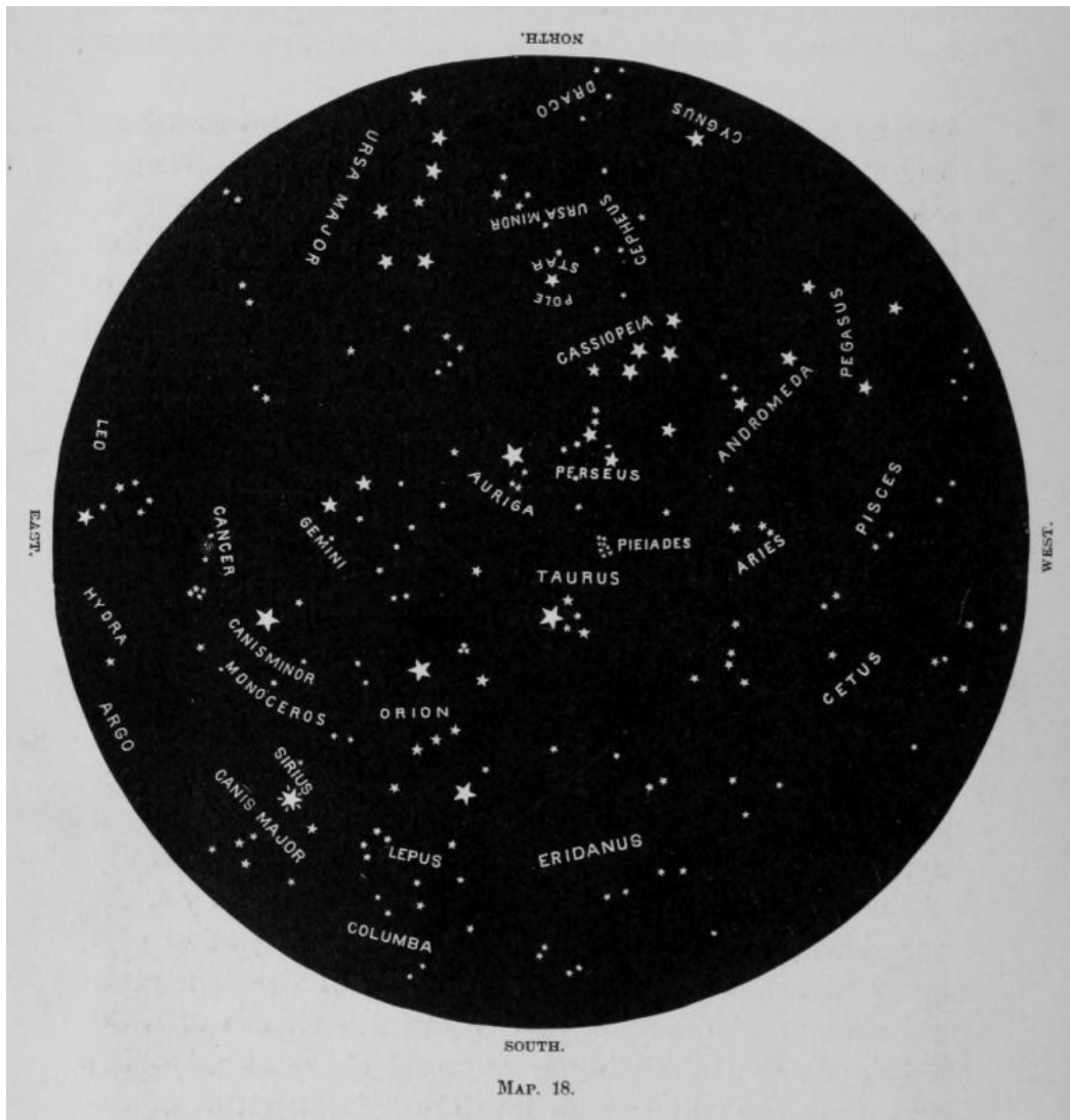
MAP. 18.
