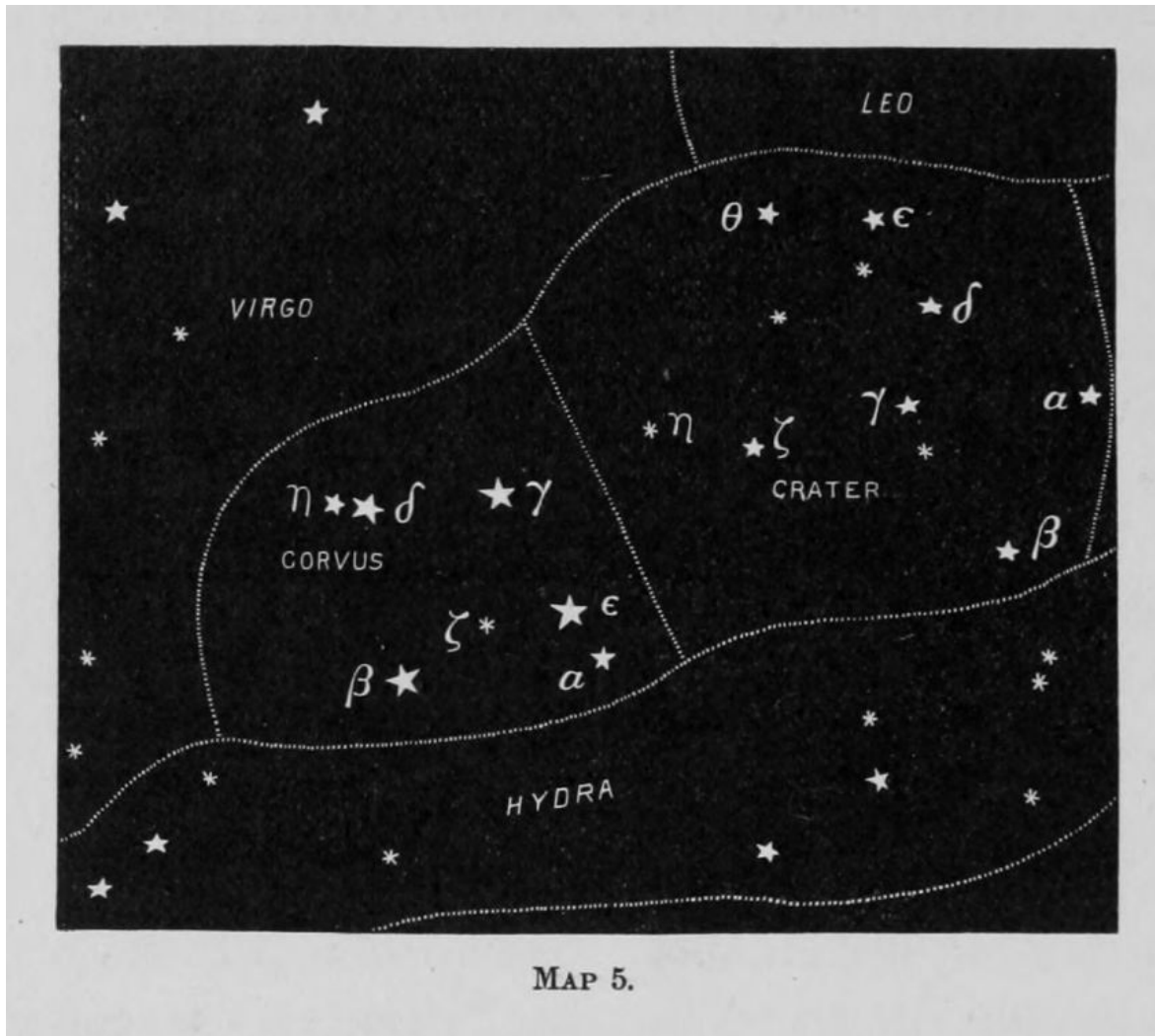
MAP 5.
