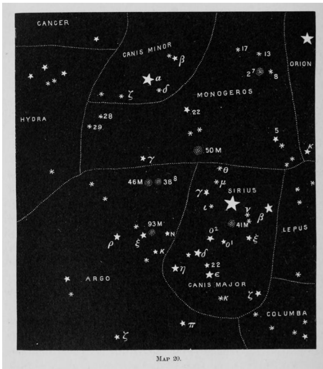
MAP 20.
