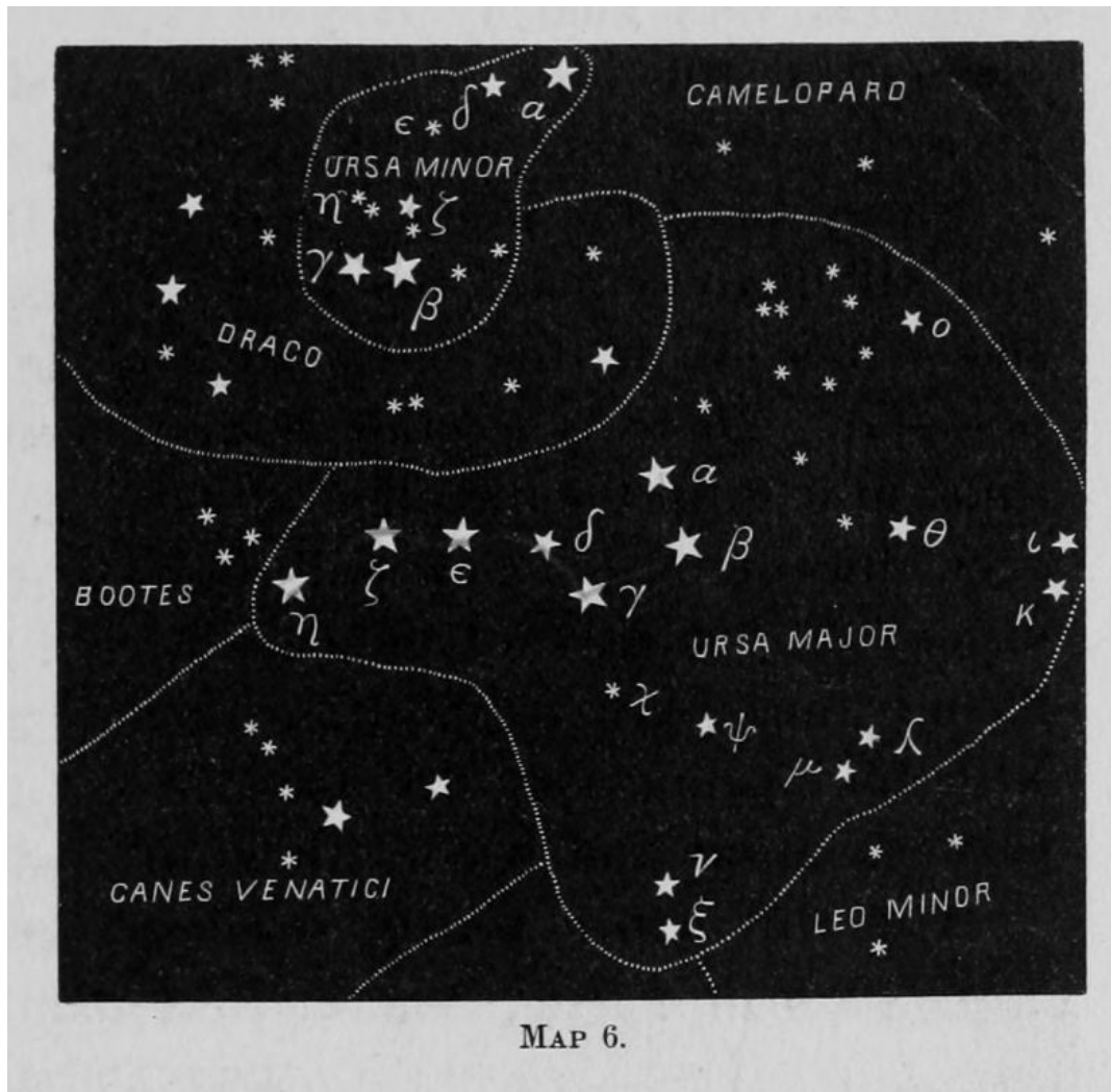
MAP 6.
