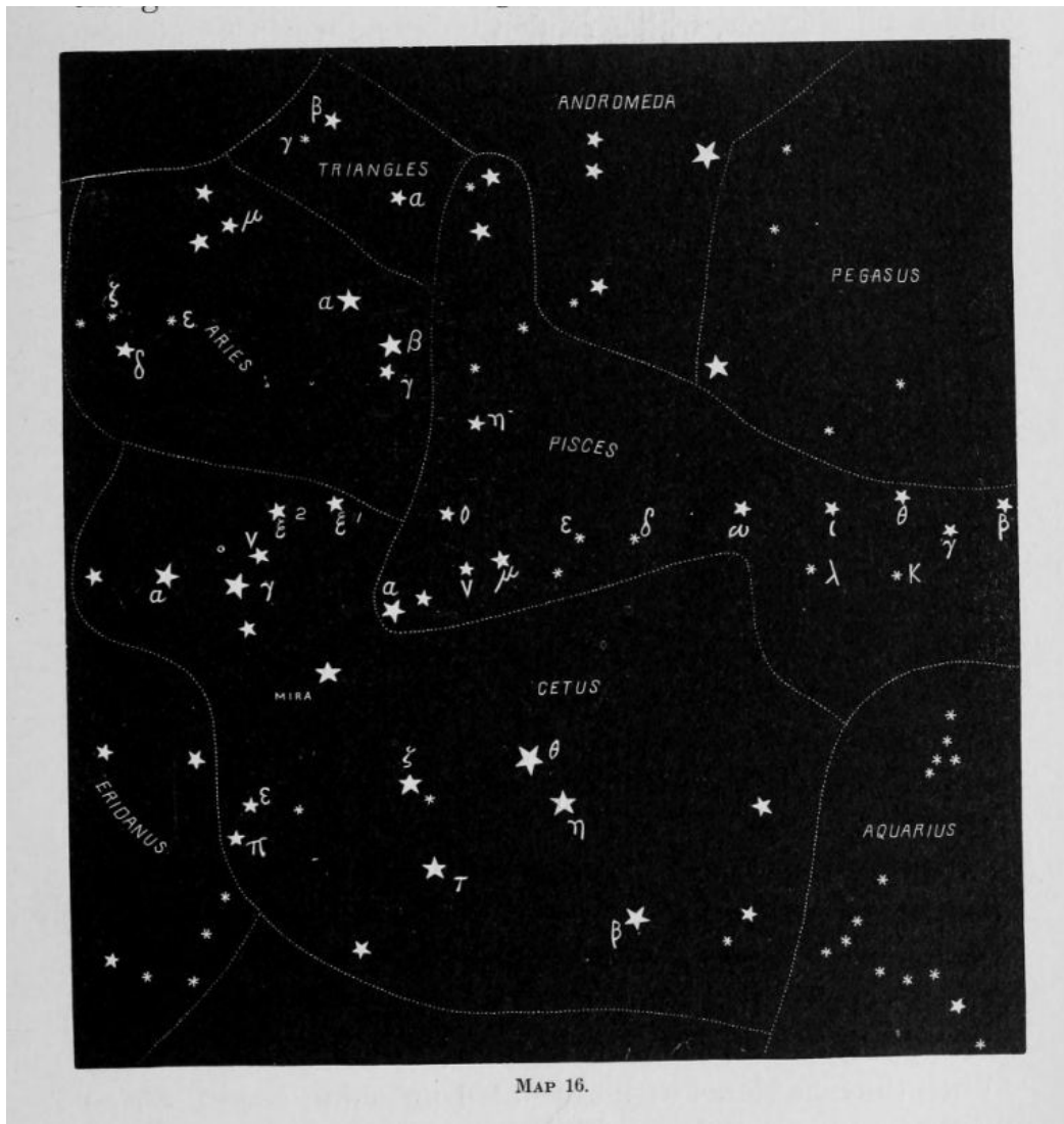
MAP 16.
