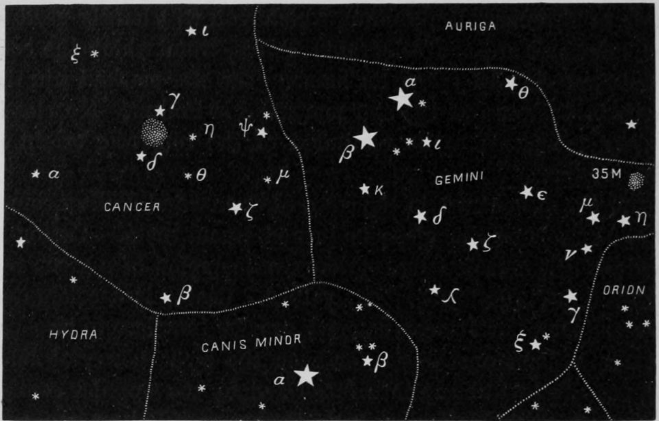
MAP 3.
