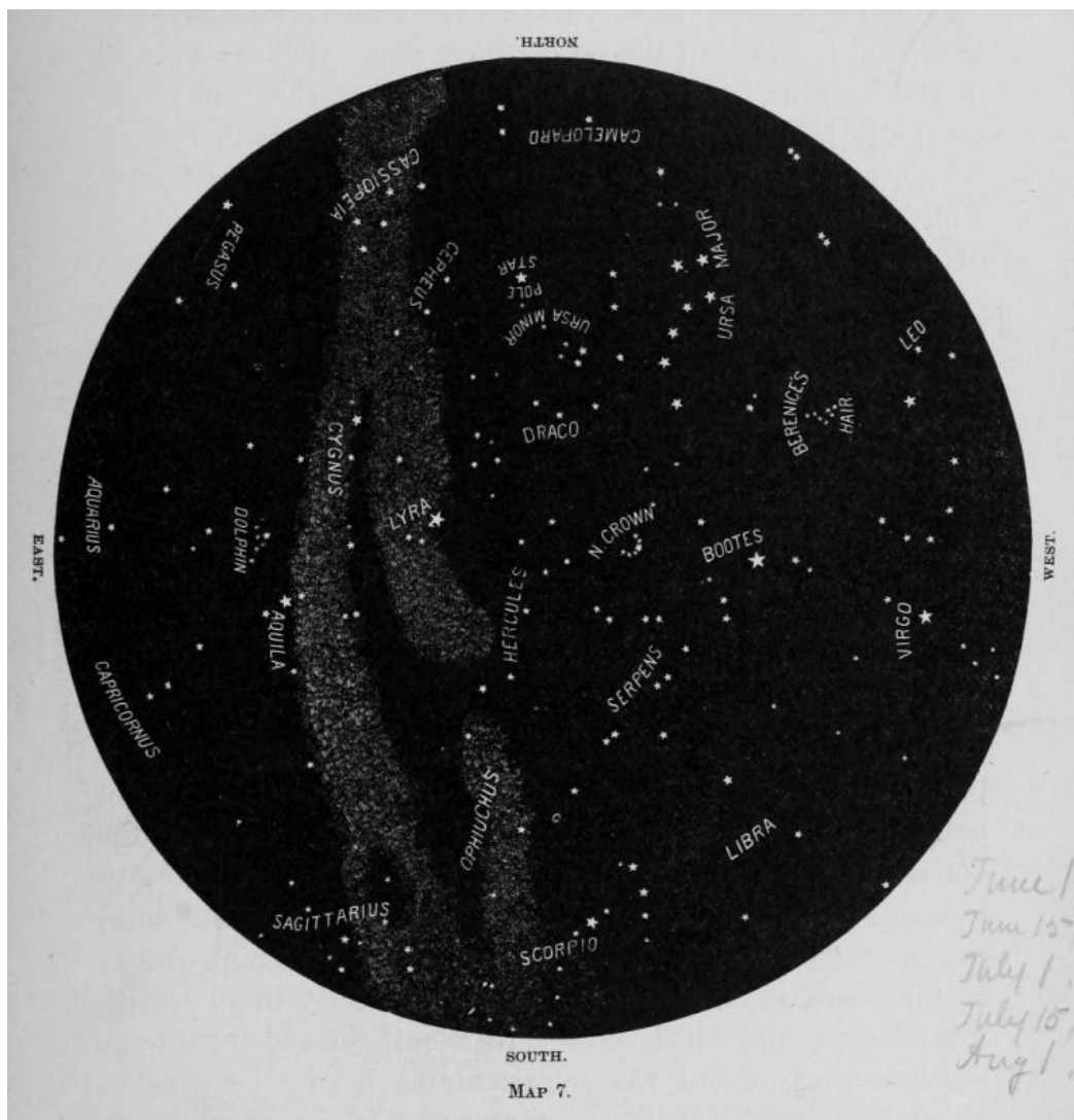
MAP 7.
