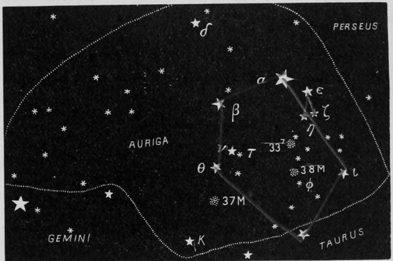
MAP 4.
