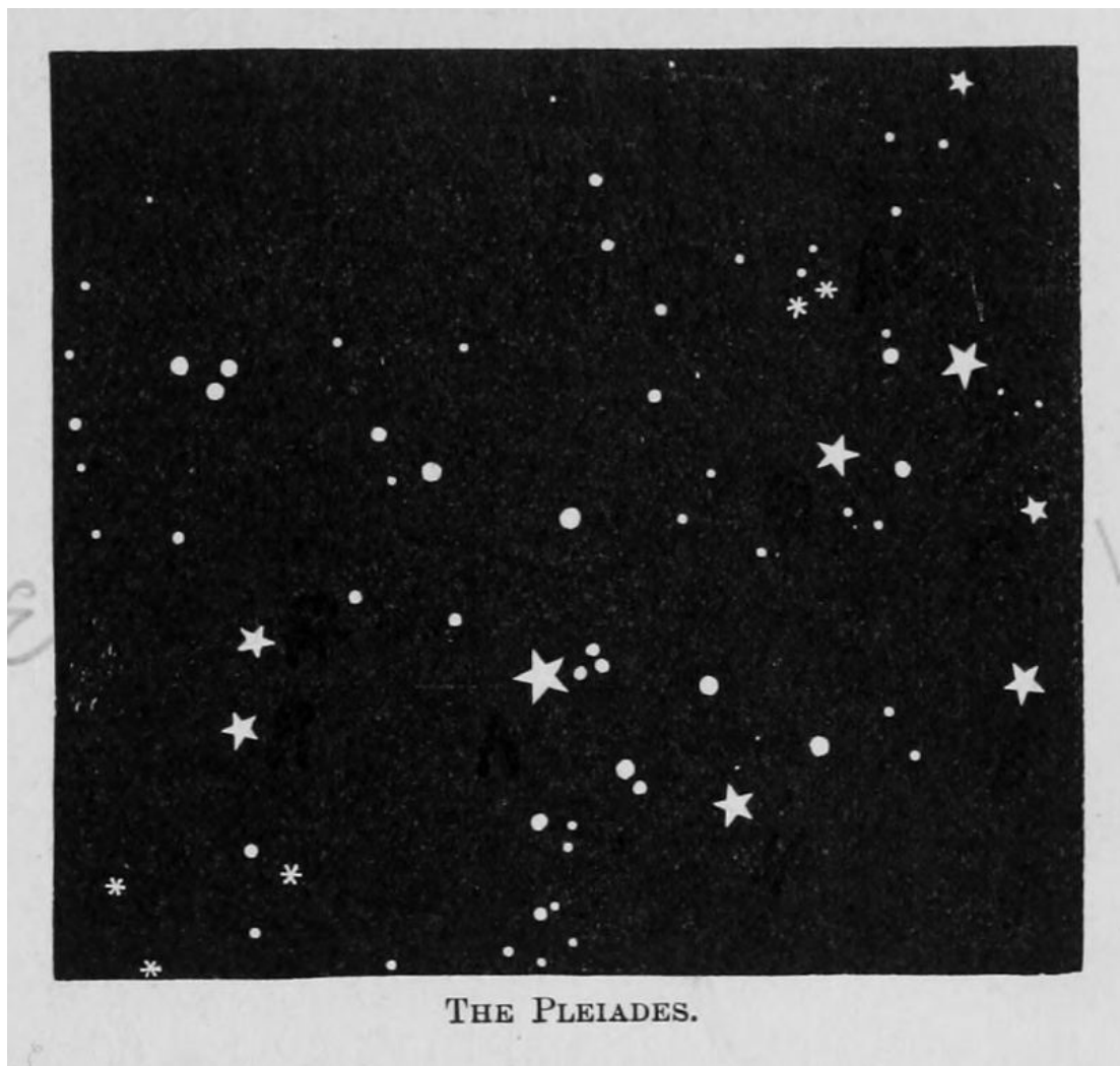
THE PLEIADES.
