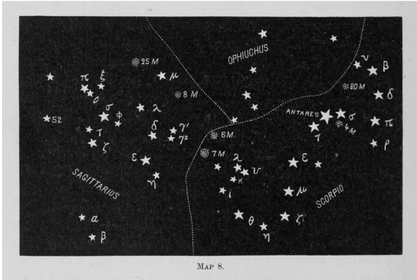
MAP 8.
