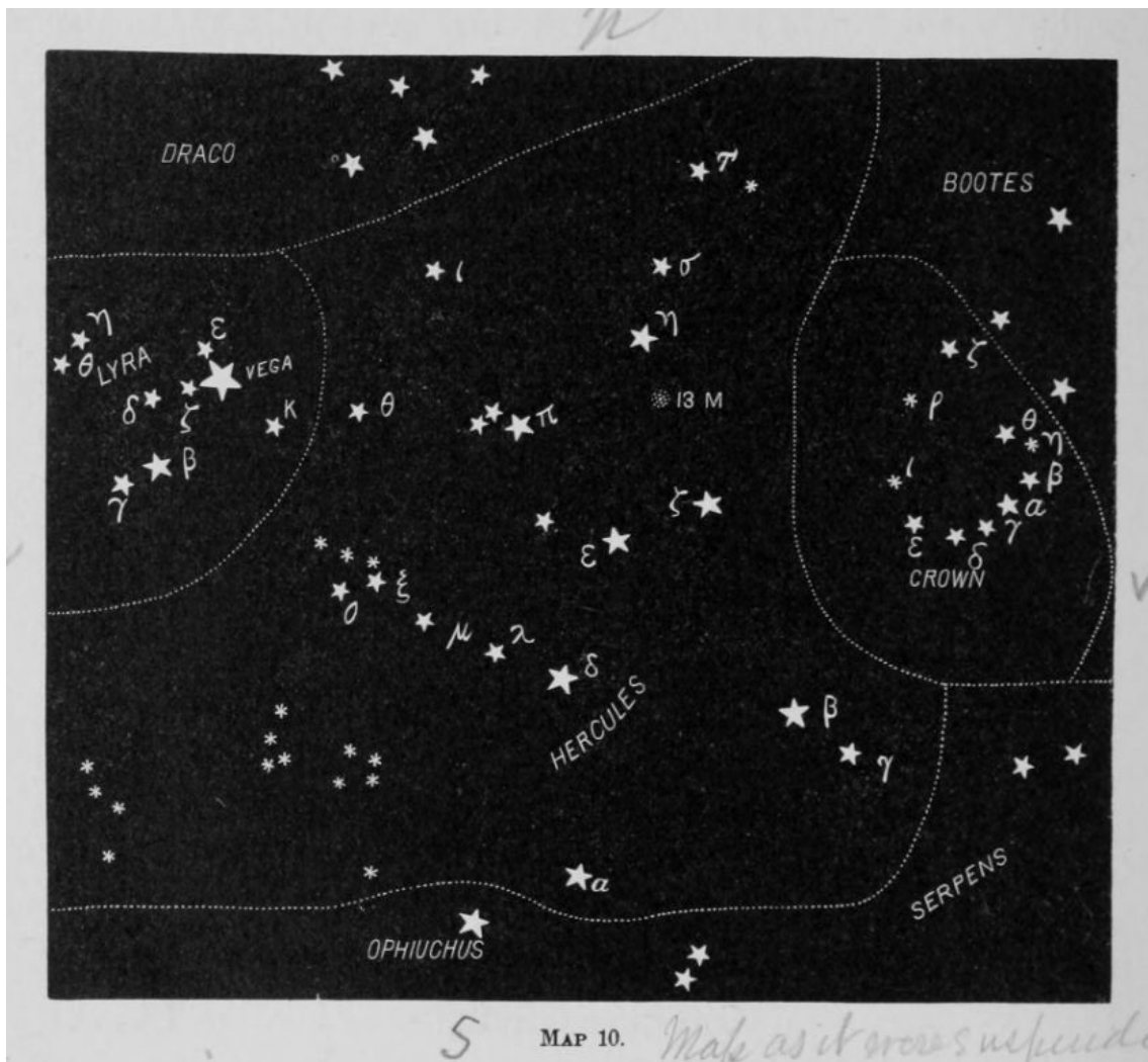
MAP 10.
