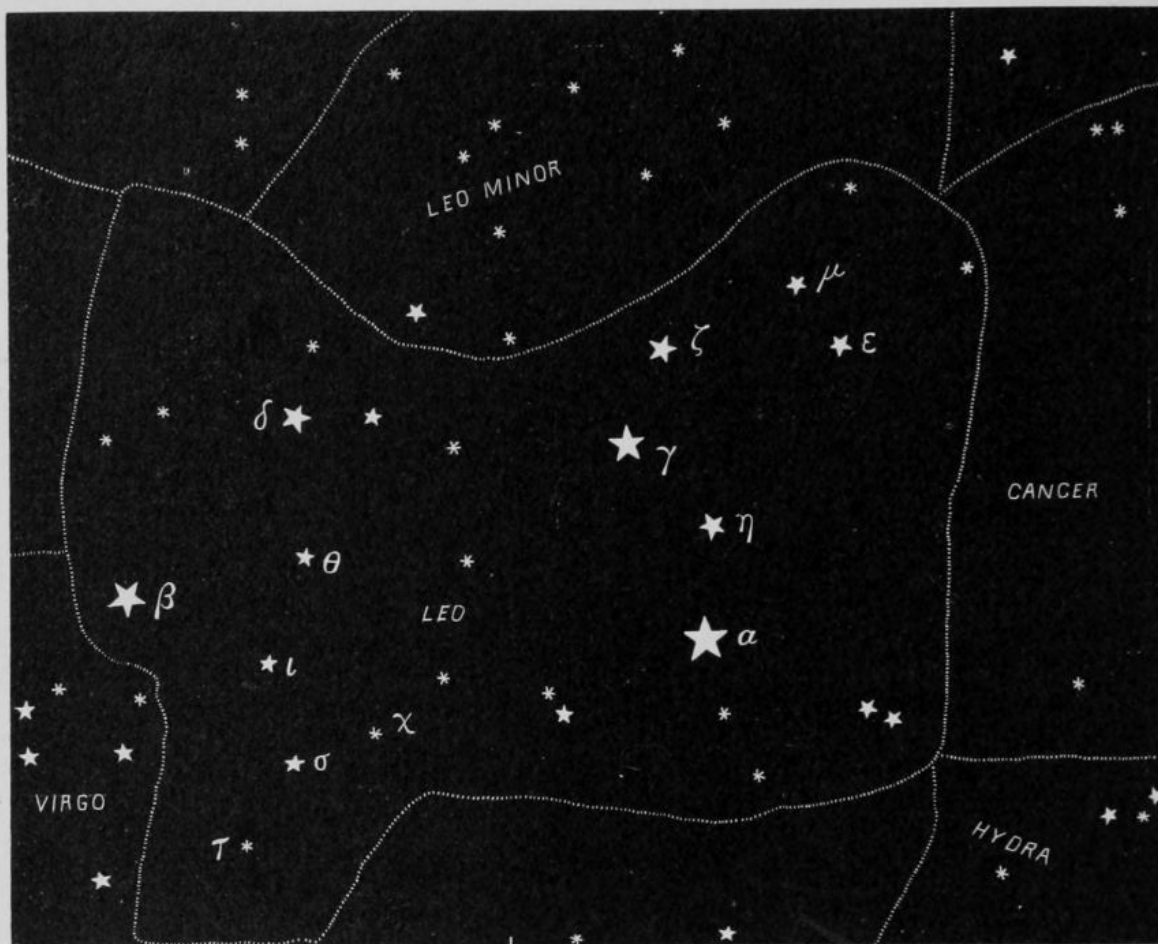
MAP 2.
