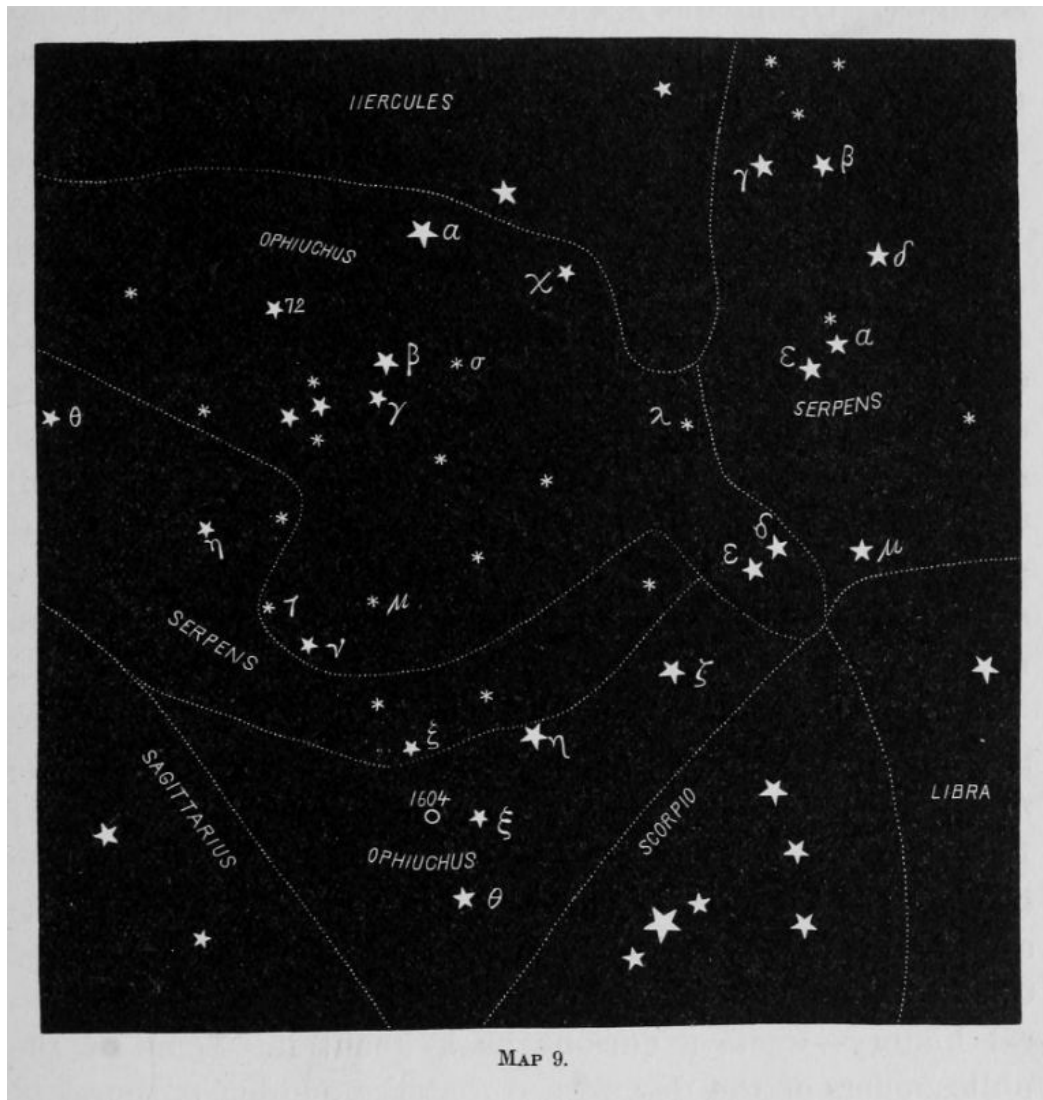
MAP 9.
