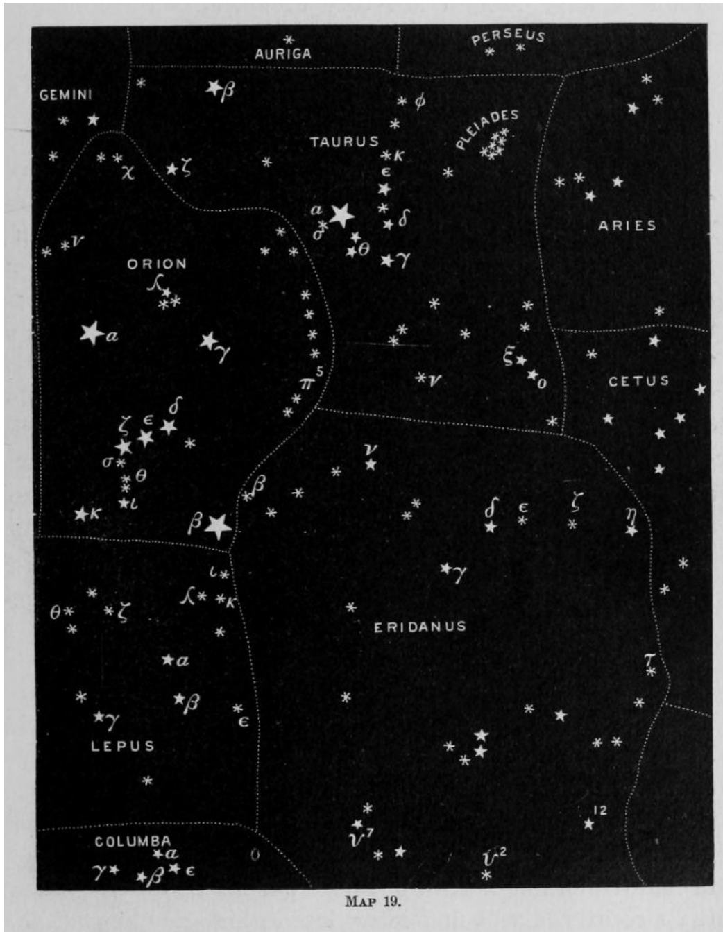
MAP 19.
