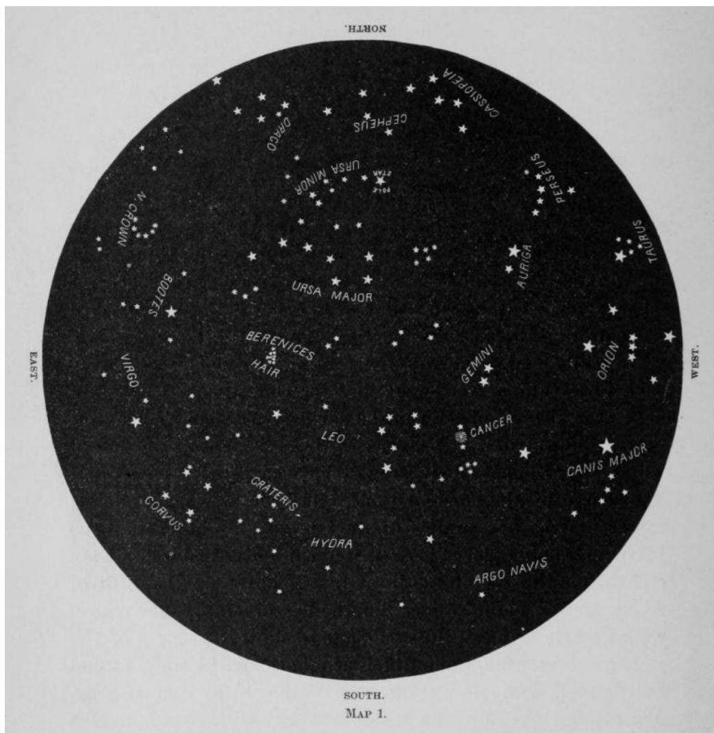
MAP 1.
