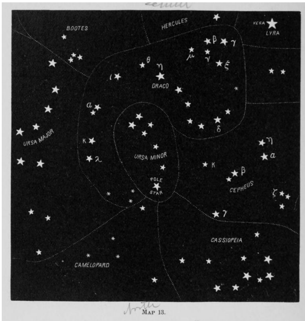
MAP 13.
