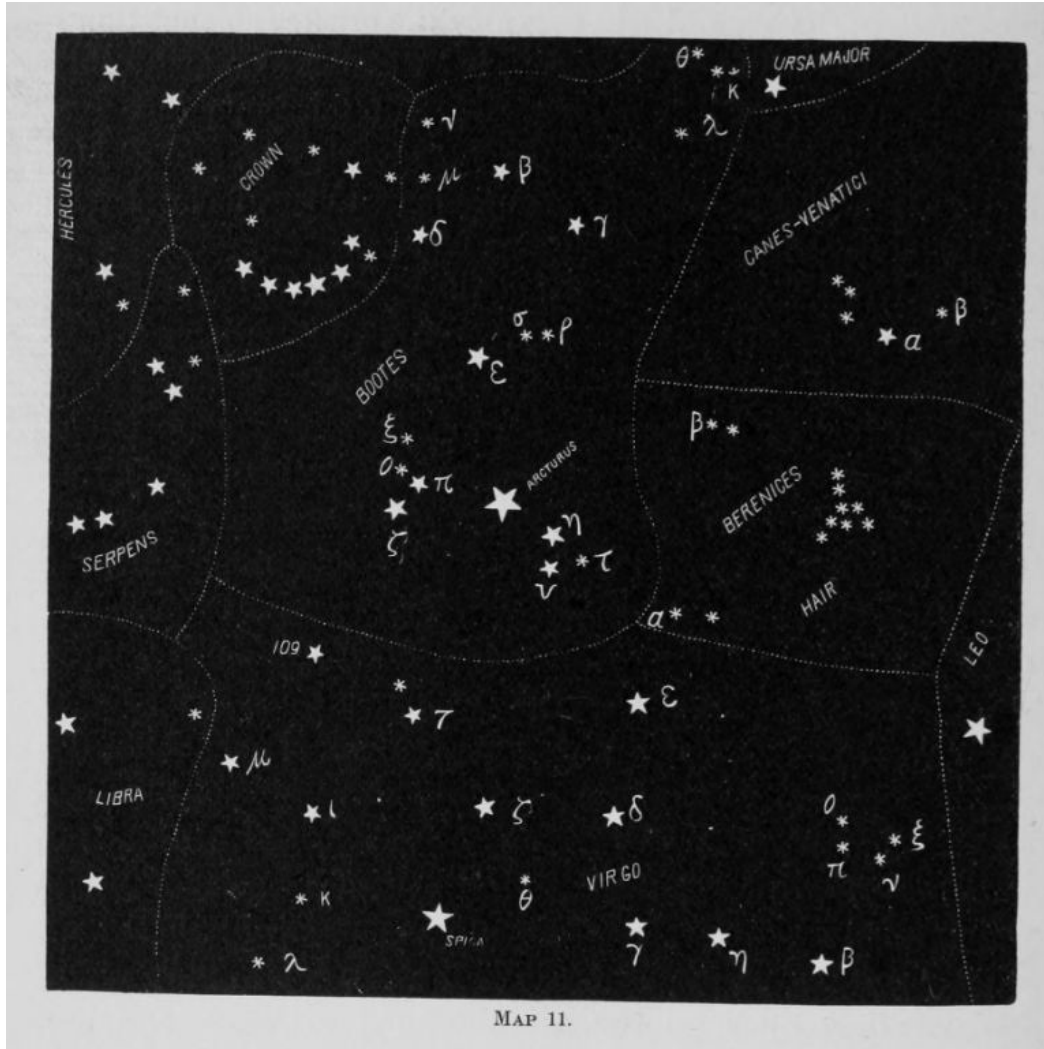
MAP 11.
