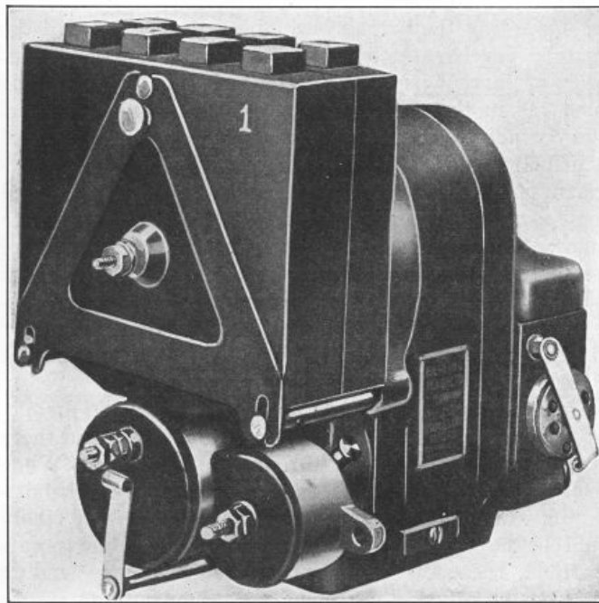
Fig. 63.—Type DD Berling High Tension Magneto.
