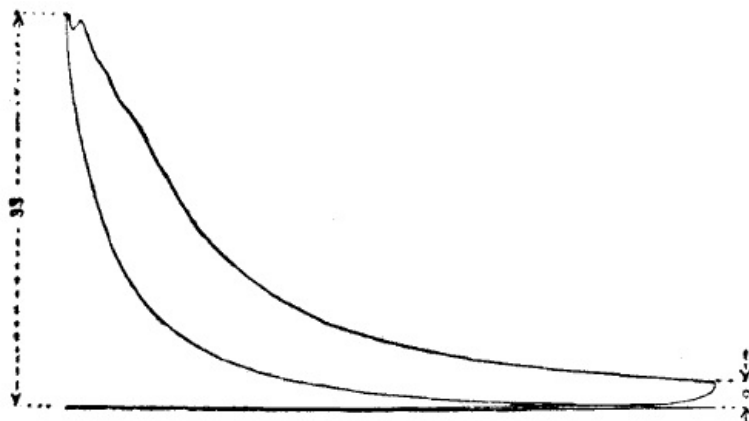
Fig. 14.—Diesel Motor Card.
