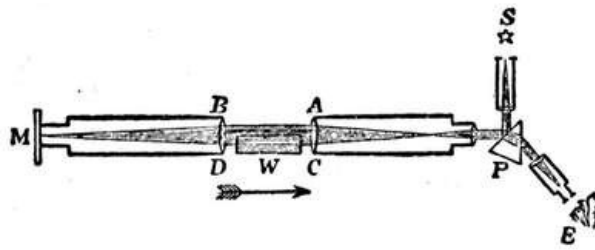
Fig. 8. Hoek's arrangement.
