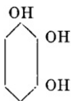
Pyrogallol.
