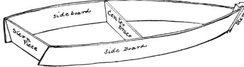
Fig. 189.—Frame.
