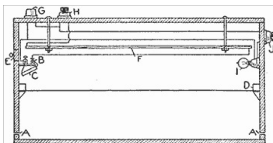
Fig. 1—Box Details
