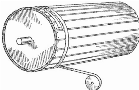
Fig. 6—Drying Reel
