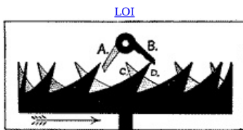
Fig. 25—Verge Escapement
