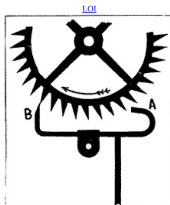
Fig. 28—American Anchor Escapement
