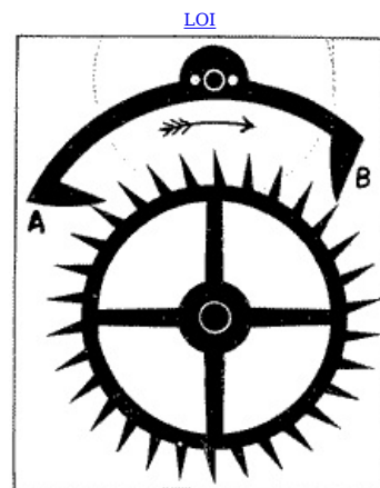
Fig. 27—Anchor Escapement
