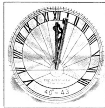
Fig. 4—12-Inch Modern Horizontal Sundial for Latitude 40°-43'
