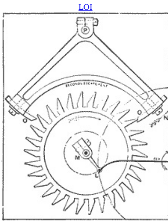
Fig. 29—Dead Beat Escapement
