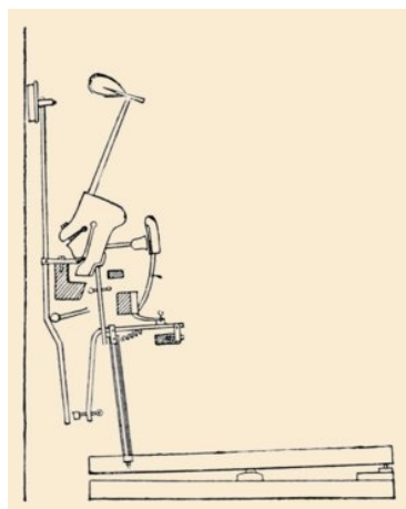
FIG. 125. MÉCANISME MODERNE DU PIANO. (Système Chickering.)
