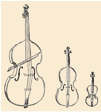
FIG. 121. CONTREBASSE.—VIOLONCELLE.—VIOLON.
