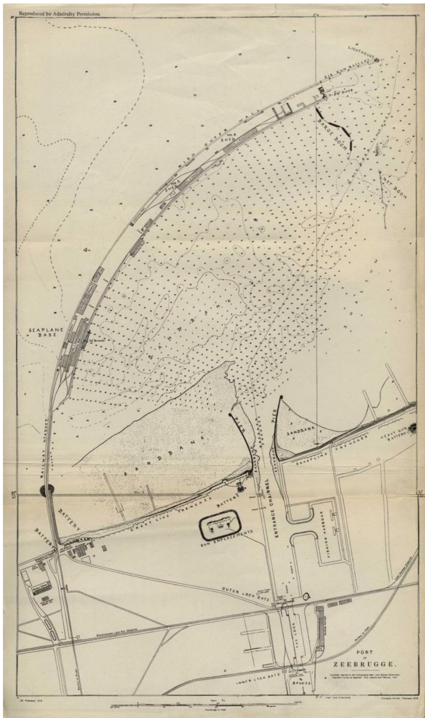
PORT OF ZEEBRUGGE
