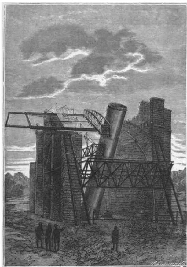
L'instrument monté. (Page 80.)
