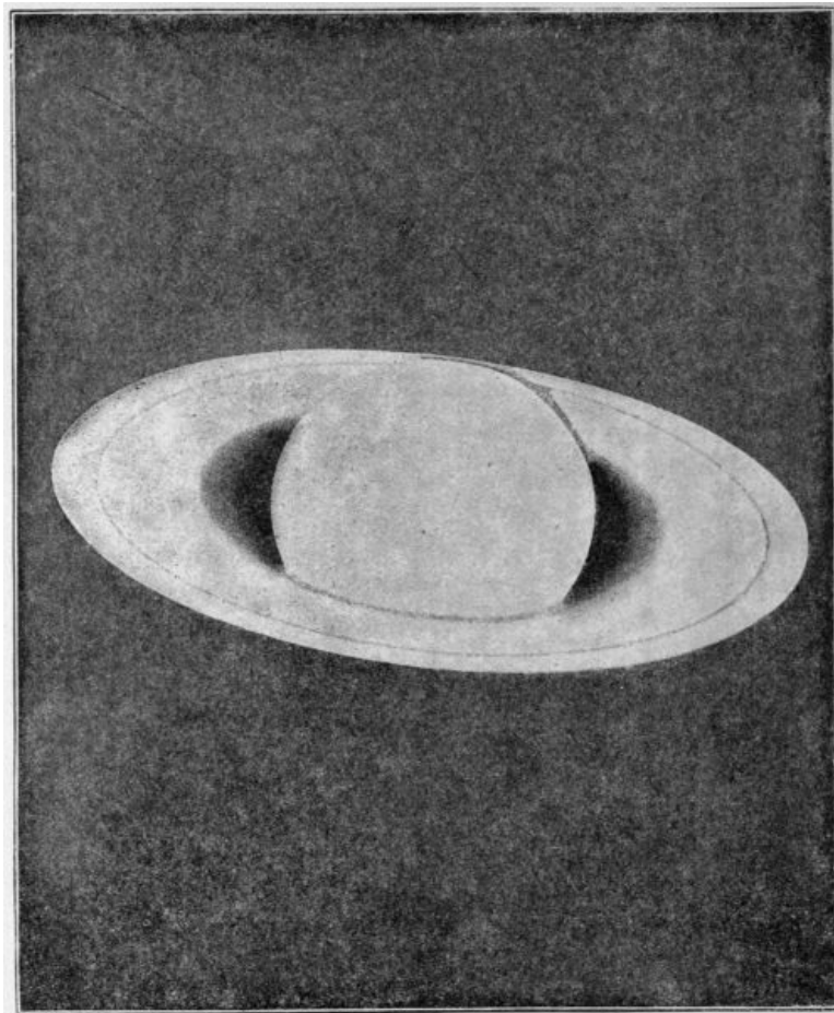
FIG. 1.—THE PLANET SATURN.
