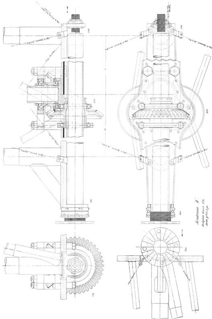
PL. 58. BEDPLATE, GEARS, ETC. ◊ lgr
