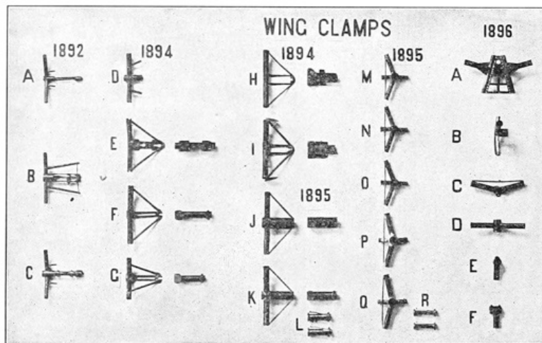
FIG. 16. Wing clamps, 1892-1896.
