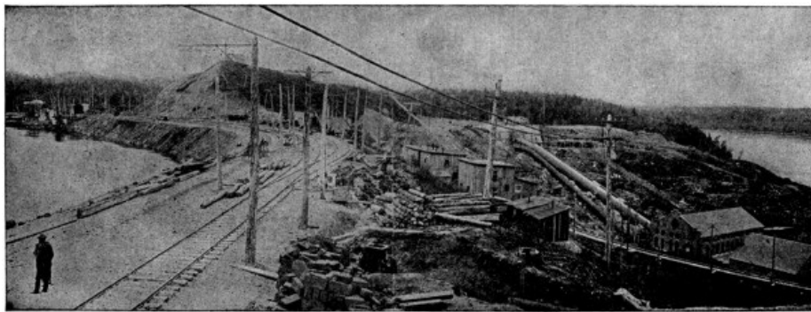
FIG. 15.—Shawinigan Falls Power-plant.
