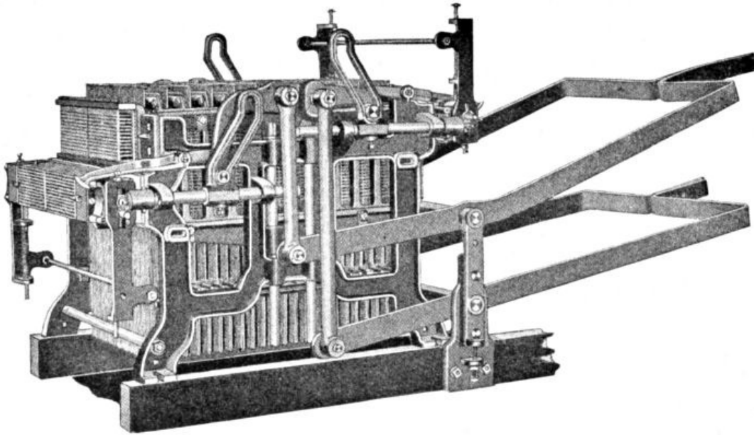
Fig. 24. Double Action Jacquard Machine.
