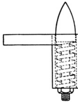
Fig. 17. Spring Peg.
