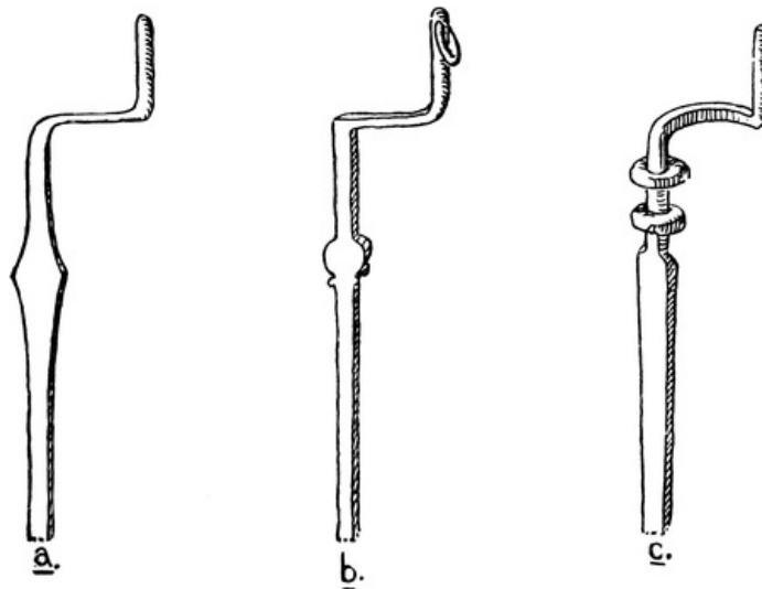
Fig. 39. a-c. Griff-Enden der Kurbelbratspieße von D., F. und G.
