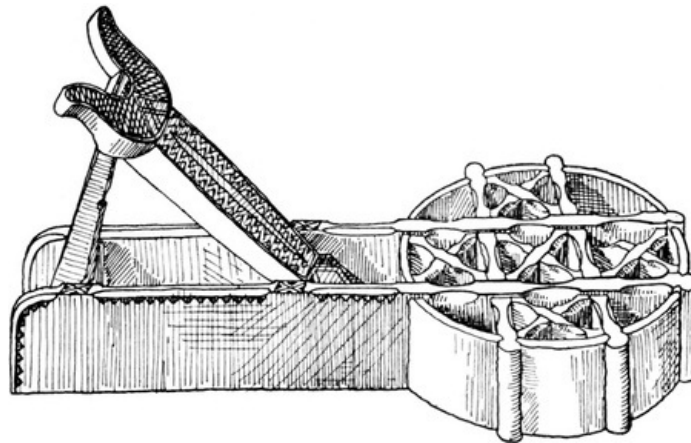
Fig. 23. Pfannenholz in der Küche des Albrecht Dürer-Hauses.
