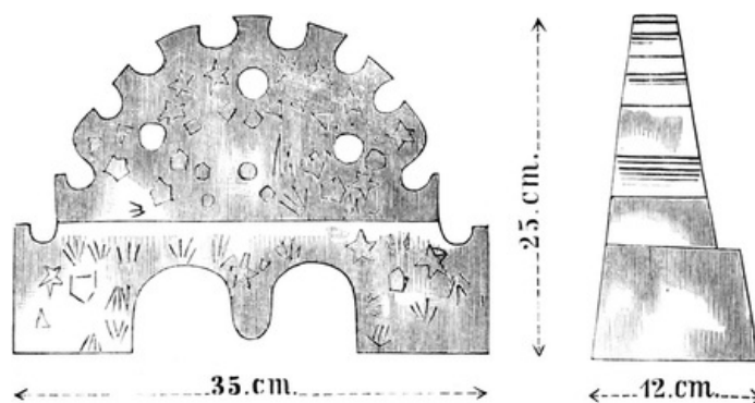
Fig. 45. Bratspießlager aus gebranntem Thone im Besitze des Museums.
