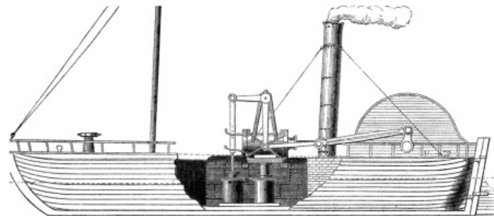
MACHINERY OF THE 'CHARLOTTE DUNDAS.'
