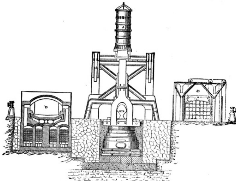
FIG. 3.--PROFILE VIEW.
