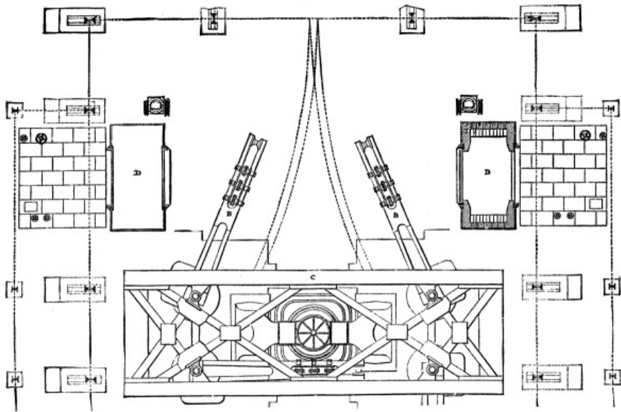
FIG. 2.--PLAN.
