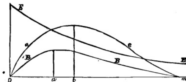
Fig. 2--KAPP'S DIAGRAM.
